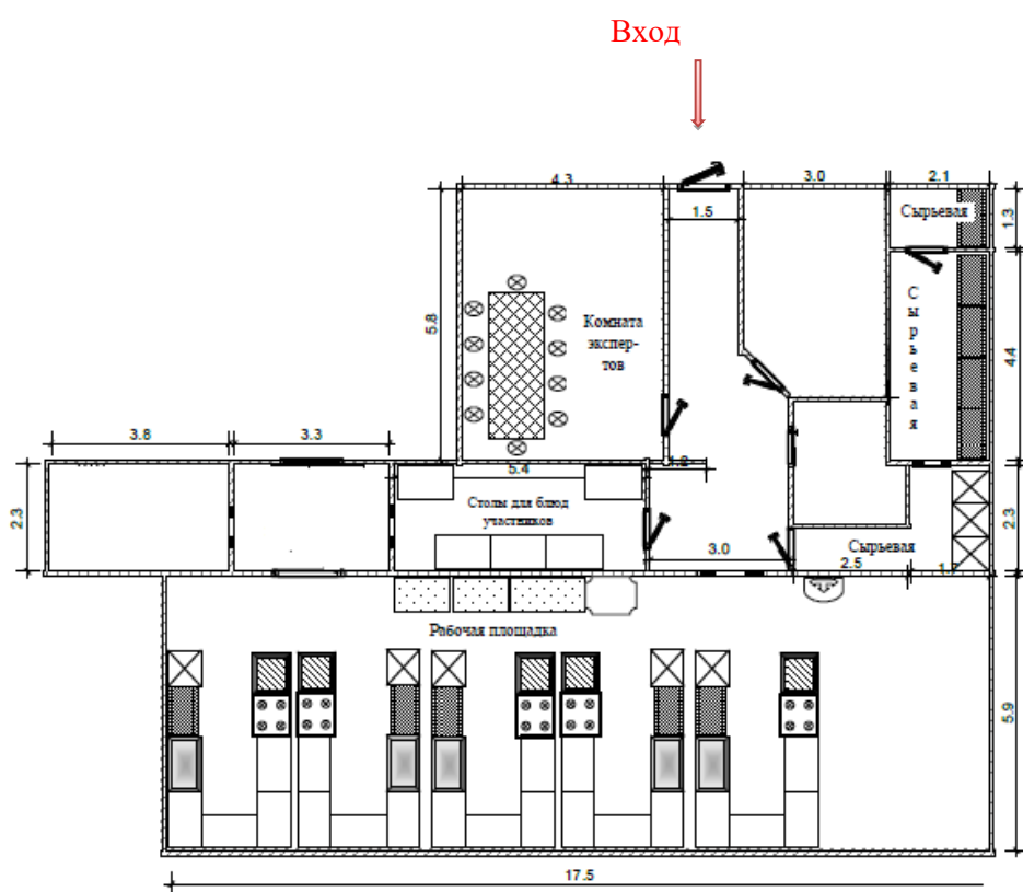
5 Схема застройки конкурсной площадки.
